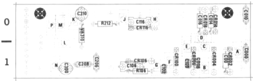
Fig. 8-2. A20 Actuator Board
